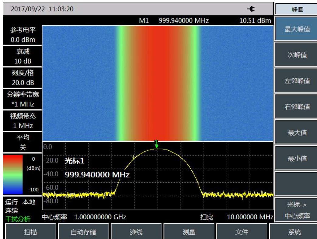
干扰分析 (瀑布图)
